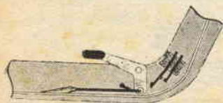
Fig. 1. — Sulla Vespa il contatto si installa al disopra del telaio. Premendo il pedale del freno, la leva mette in contatto le due lamelle d'ottone, chiudendo così il circuito.
