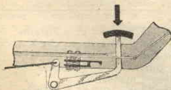
Fig. 2. — Sulla Lambretta invece, il contatto si installa sotto il telaio, ed è sistemato in modo, che una lamella di ottone viene tenuta sollevata. Premendo sul pedale del freno, le due lamelle vengono in contatto.
