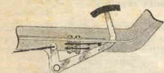
Fig. 1. — Sulla Vespa il contatto si installa al disopra del telaio. Premendo il pedale del freno, la leva mette in contatto le due lamelle d'ottone, chiudendo così il circuito.
