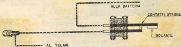
Fig. 4. — Un impianto a portalampada non isolato richiede un impianto così modificato e un isolante sulla lamella mobile, per evitare che questa venga a contatto con la leva del freno; poiché in questo caso, si avrebbe inevitabilmente un cortocircuito.
