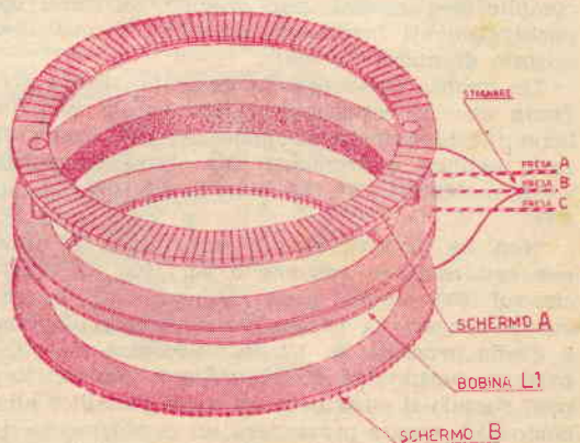
Fig. 6. — La bobina oscillatrice L1 dovrà essere disposta entro ai due schermi A e B come mostra la figura.
