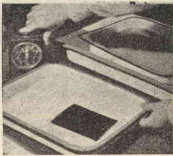
Fig. 6. - Tolta la fotografia dal bagno di sviluppo, la s'immerge per 2 minuti in una seconda bacinella contenente il bagno d'arresto.
