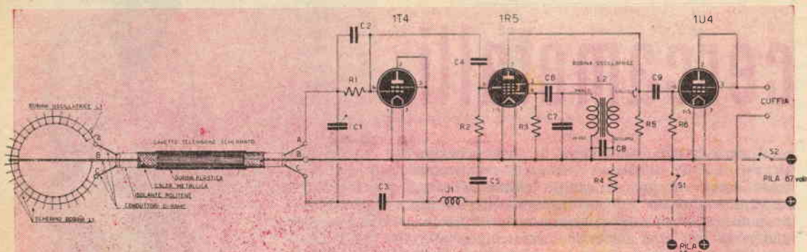
Fig. 1. — SCHEMA ELETTRICO. VALORE E PREZZO DEI COMPONENTI:
