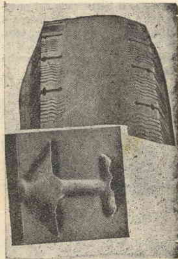
Fig. 7. — Usura dei pneumatici anteriori.
